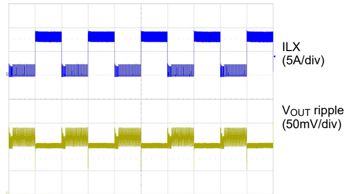
Load Transient 0A to 8A
